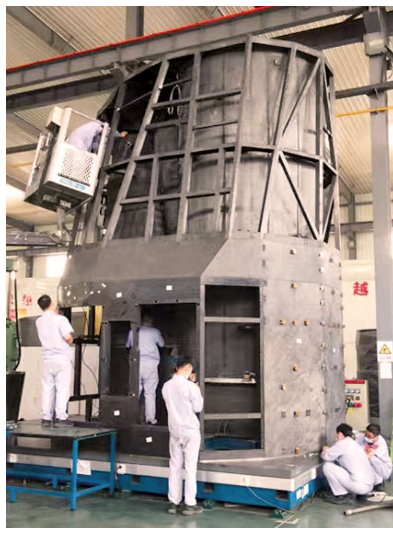
2021年王维和团队成员在望远镜结构组装现场
