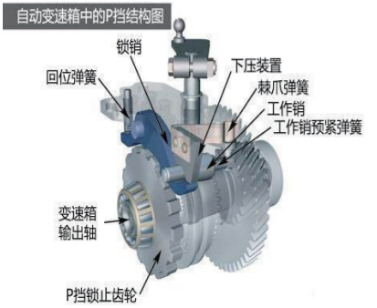
自动挡变速箱中的P挡结构图
