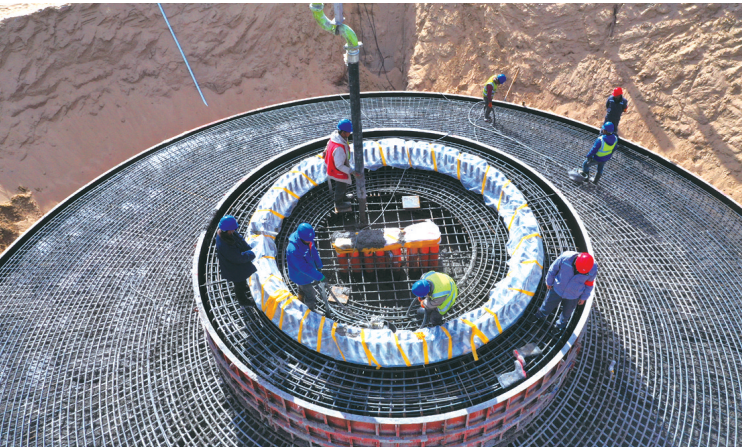
奈曼旗明阳智慧能源30万千瓦风电项目建设现场。王阳 摄
