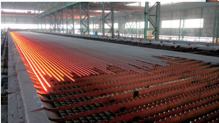
轧钢厂冷床。毕力格 摄
