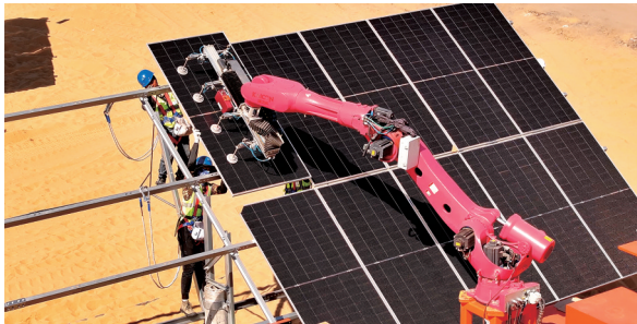
在“阿电入乌”区域互济新能源项目沙漠腹地，“光伏智能铺装机器人”正在进行铺装作业。
