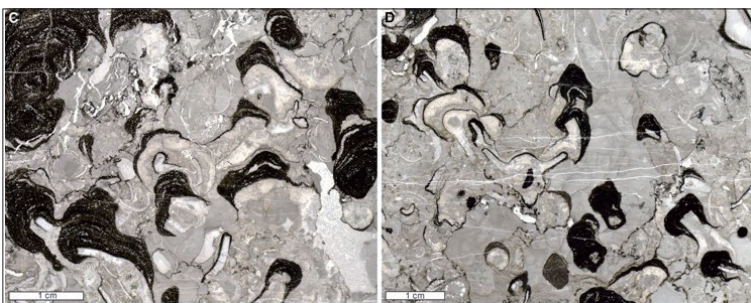
此次研究发现的层孔海绵-棘皮动物生物礁
