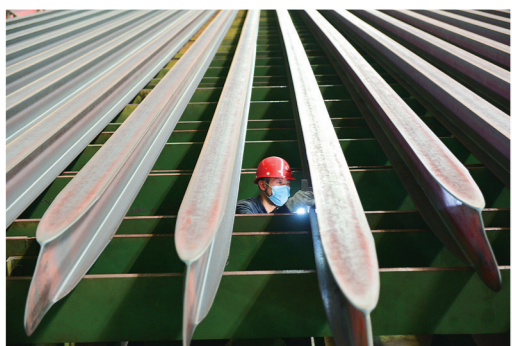
包钢集团生产的500米轨H型钢。
