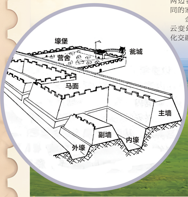
金界壕的建筑结构与功能示意图
